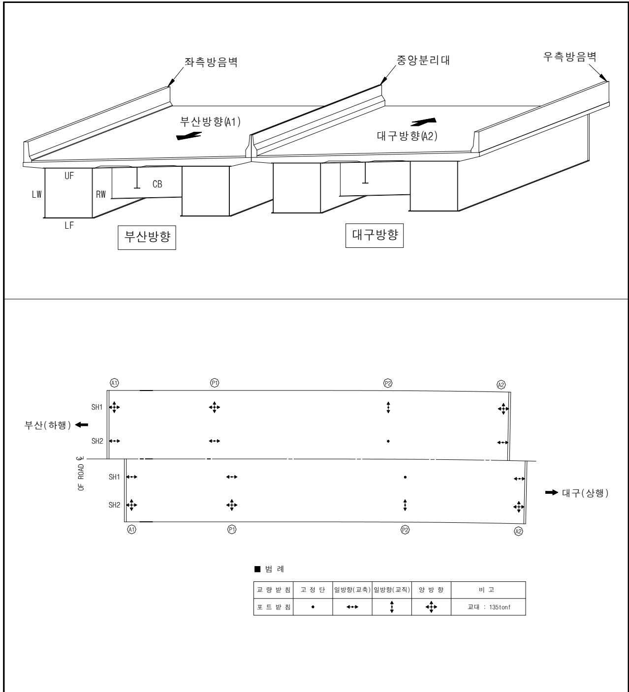
【그림 1.4.5】 교량기호의 정의
