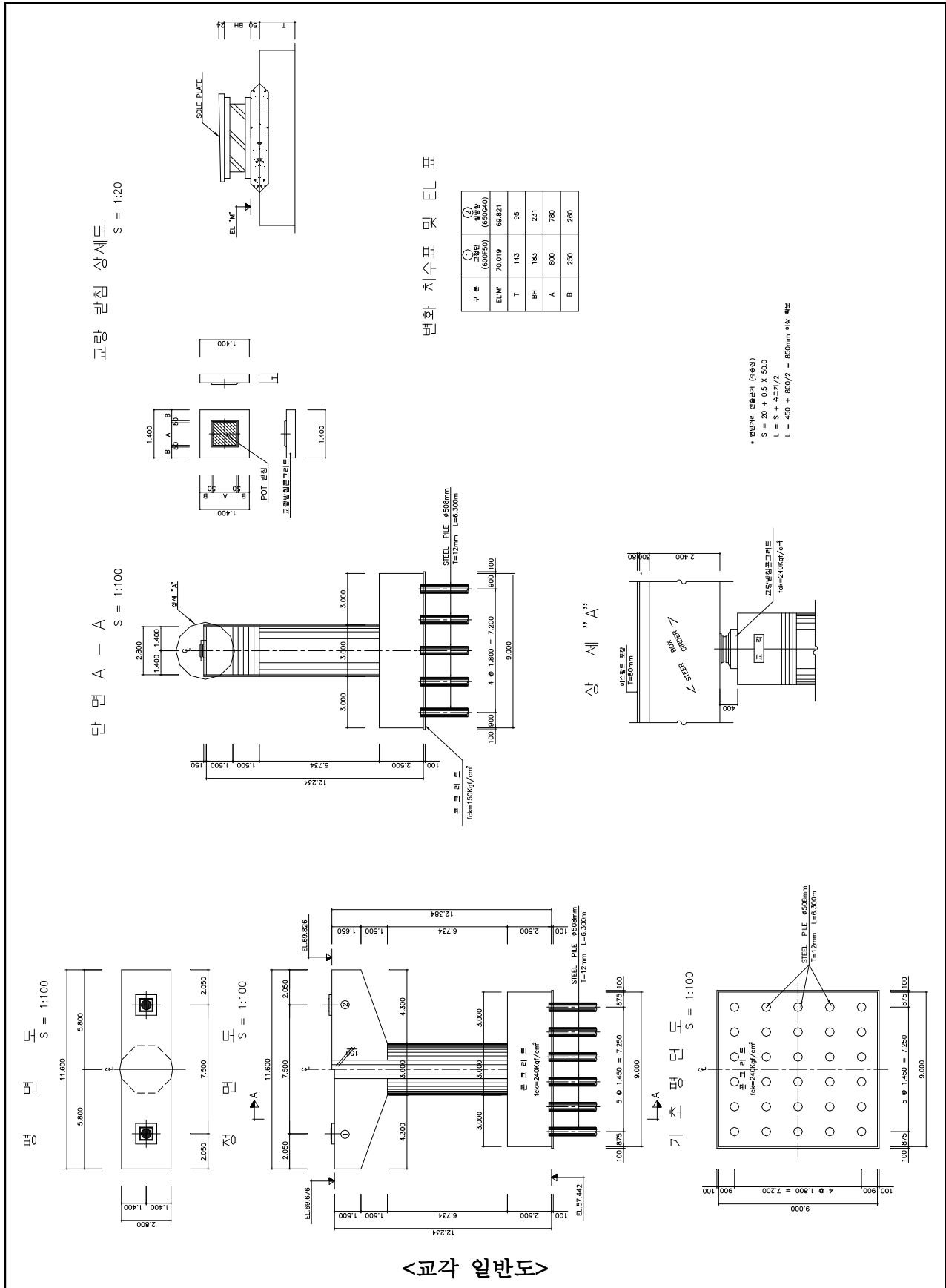
【그림 14.4】 원정교 교각 일반도
