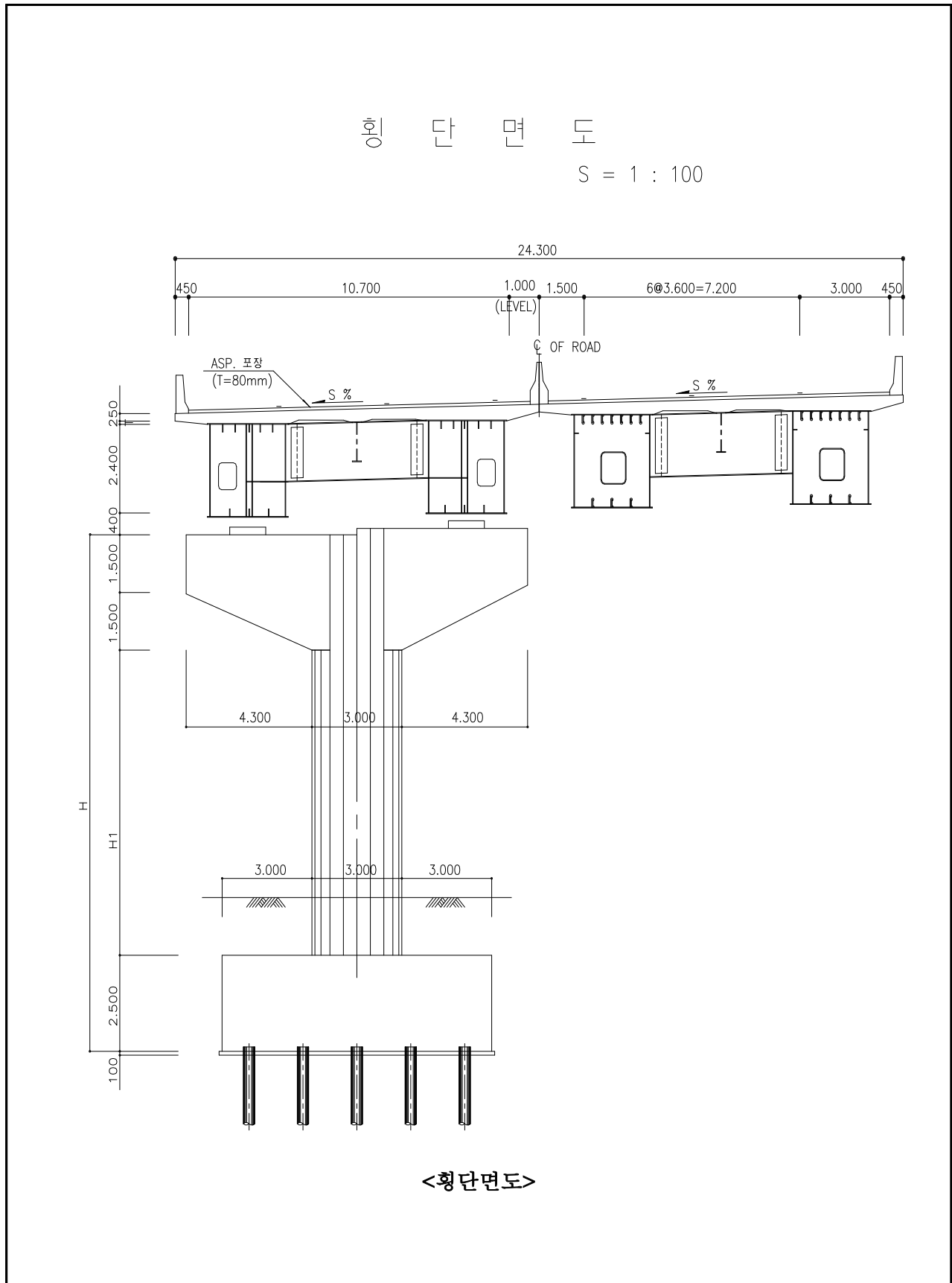
【그림 1.4.2】 원정교 횡단면도
